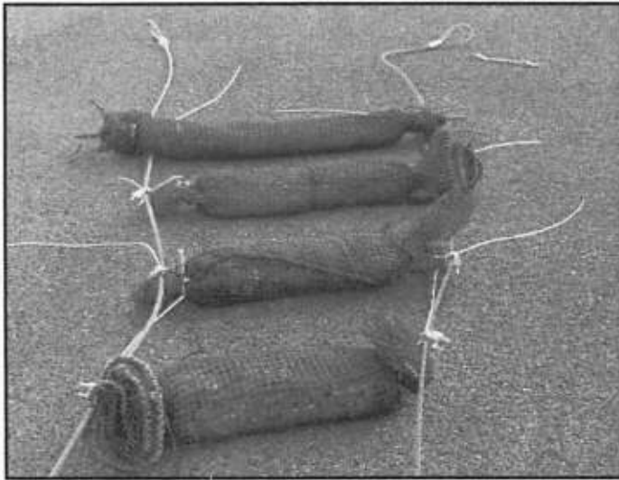
写真2：縄ばしご型魚道
